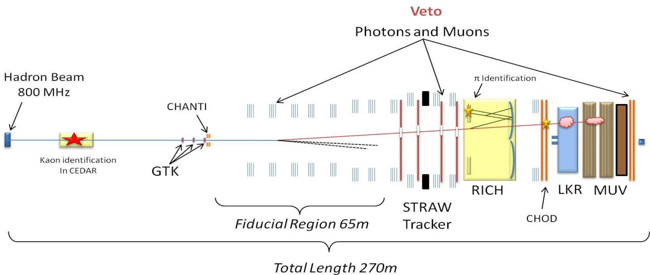
Рис. 3. Схематическое изображение экспериментальной установки NA62.
